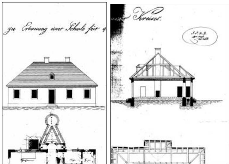
Fig.2. Planul școlii din Ciudei (1837)
